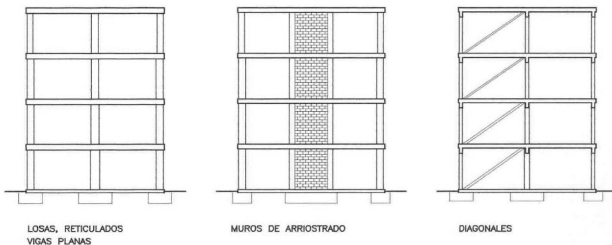
Figura 3.6.- Ejemplos de organizaciones estructurales que permiten un valor del coeficiente de comportamiento por ductilidad \mu = 2 .
