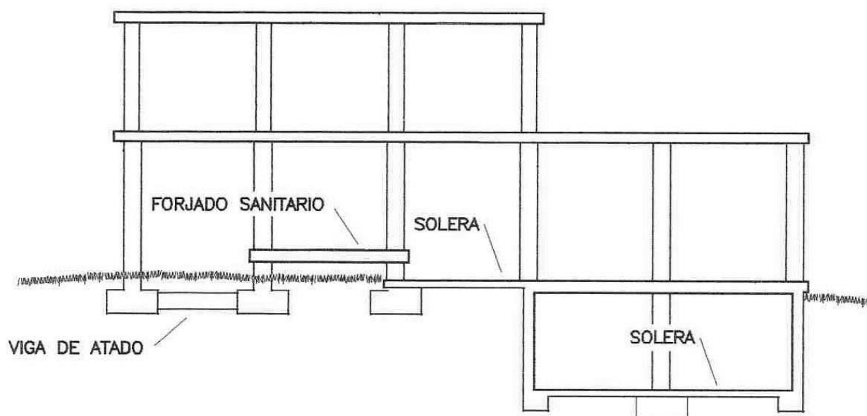
Figura 4.3. Disposición de elementos de atado.
