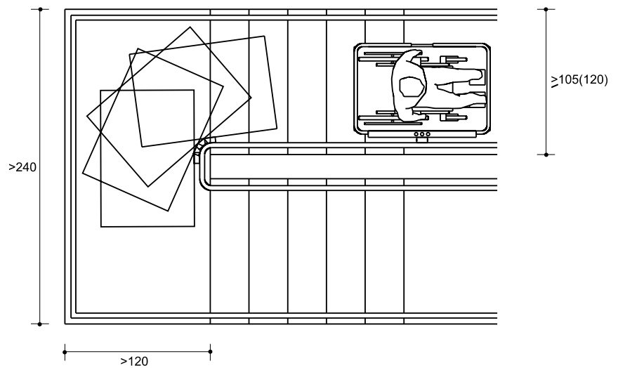
Figura 32.- Plataforma salvaescaleras en dos tramos con giro. Cotas en cm
