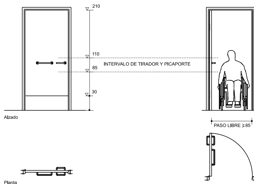
Figura 64.- Puertas abatibles. Cotas en cm
