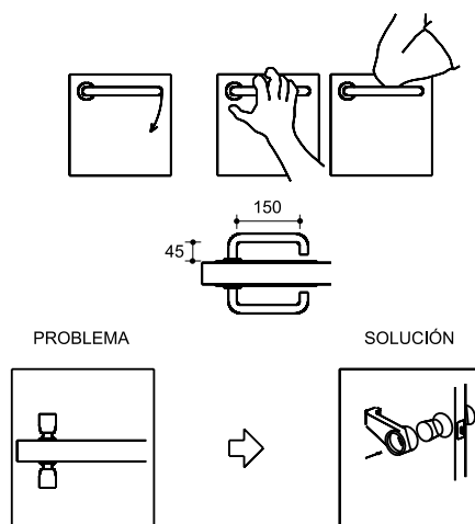
Figura 72.- Manillas. Cotas en cm
