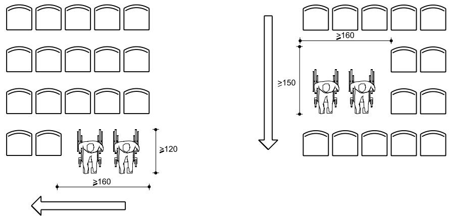
Figura 36.- Salas de reunión y espectáculos. Condiciones espaciales. Cotas en cm
