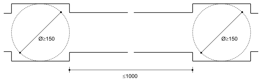
Figura 18.- Pasillos: espacios de giro. Cotas en cm
