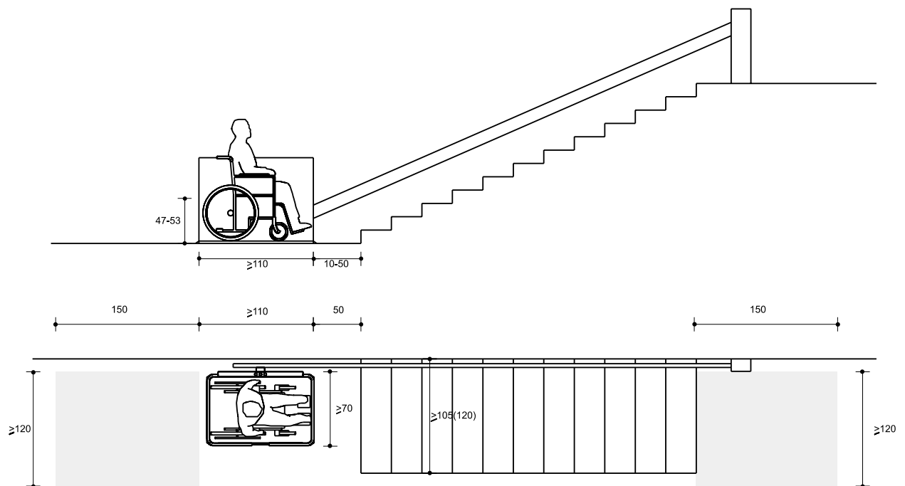
Figura 33.- Plataforma salvaescaleras en tramos rectos. Cotas en cm
