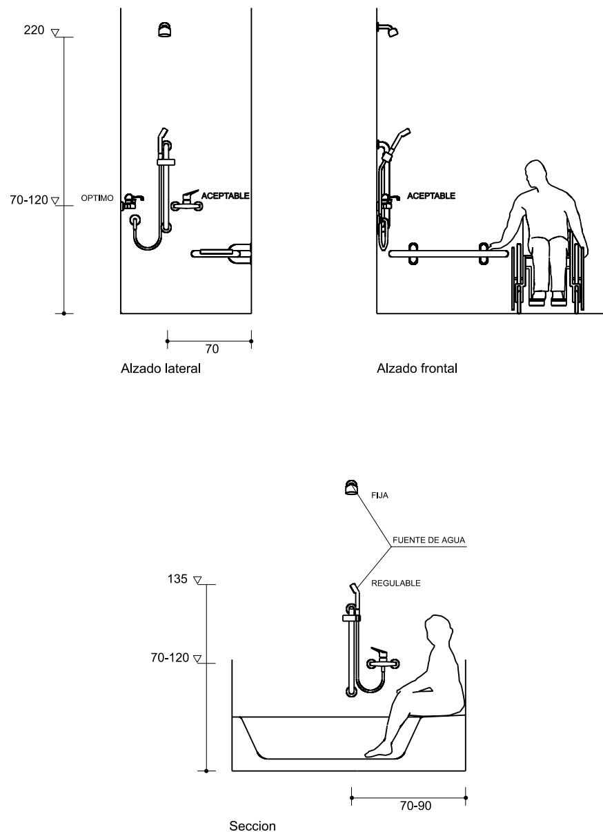
Figura 52.- Grifería. Control y fuente de agua. Cotas en cm
