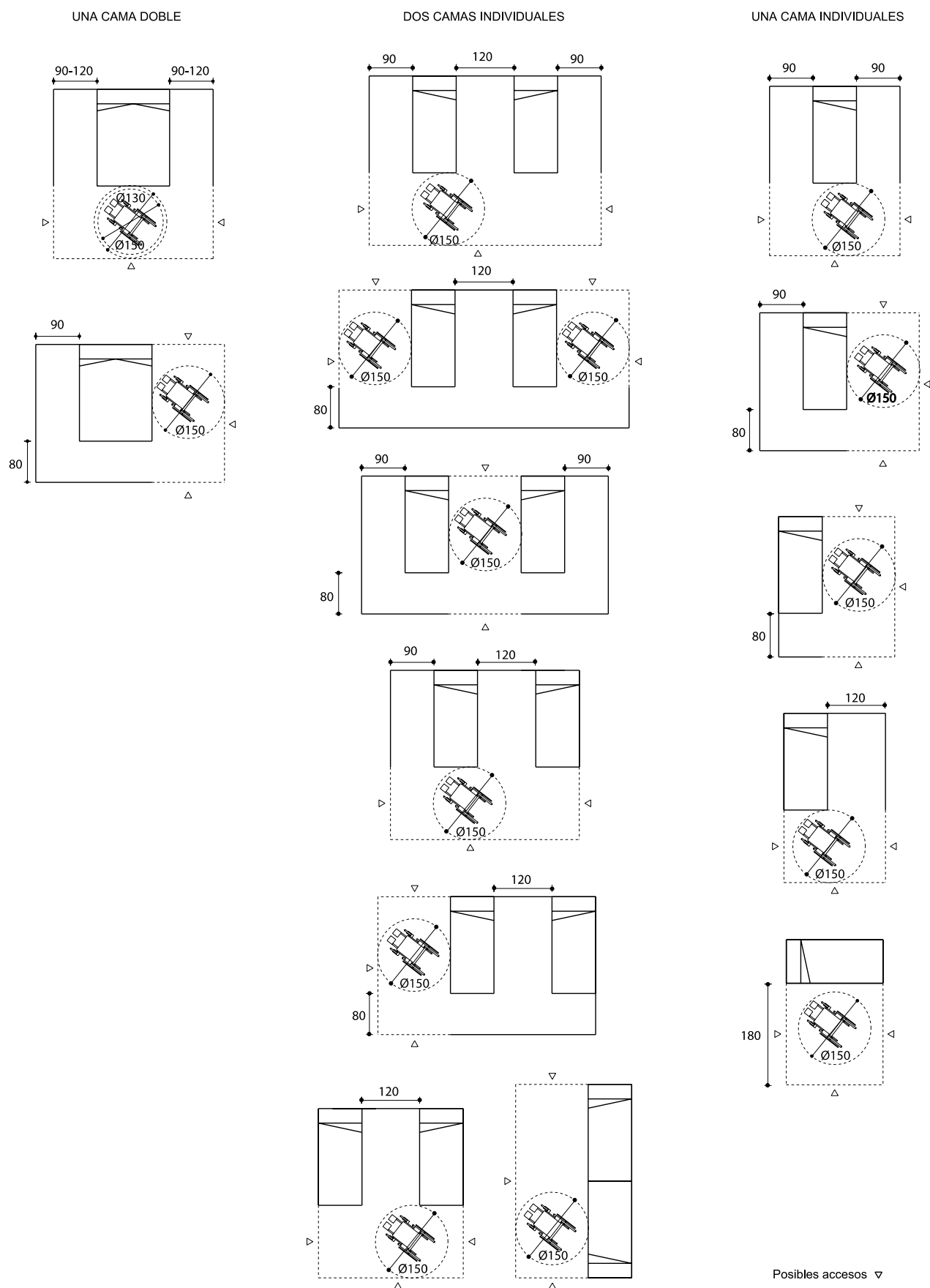
Figura 38.- Dormitorios. Espacios de uso mínimo según transferencia a la cama. Cotas en cm
