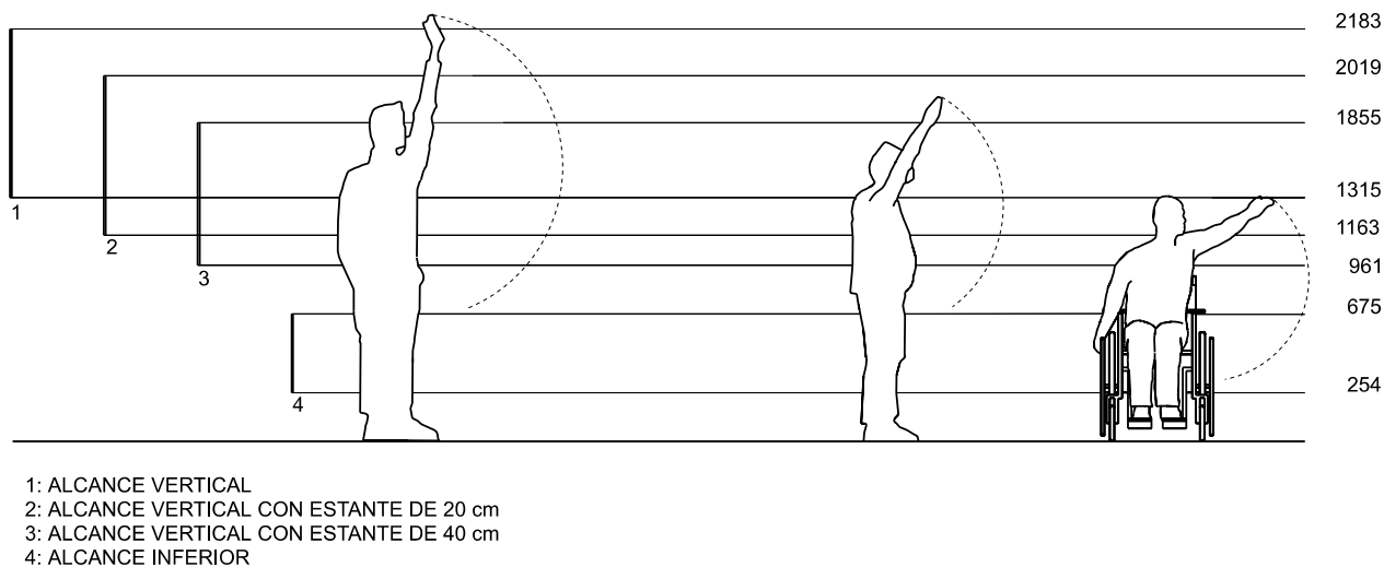
Figura 6.- Dimensiones antropométricas. Cotas en mm
