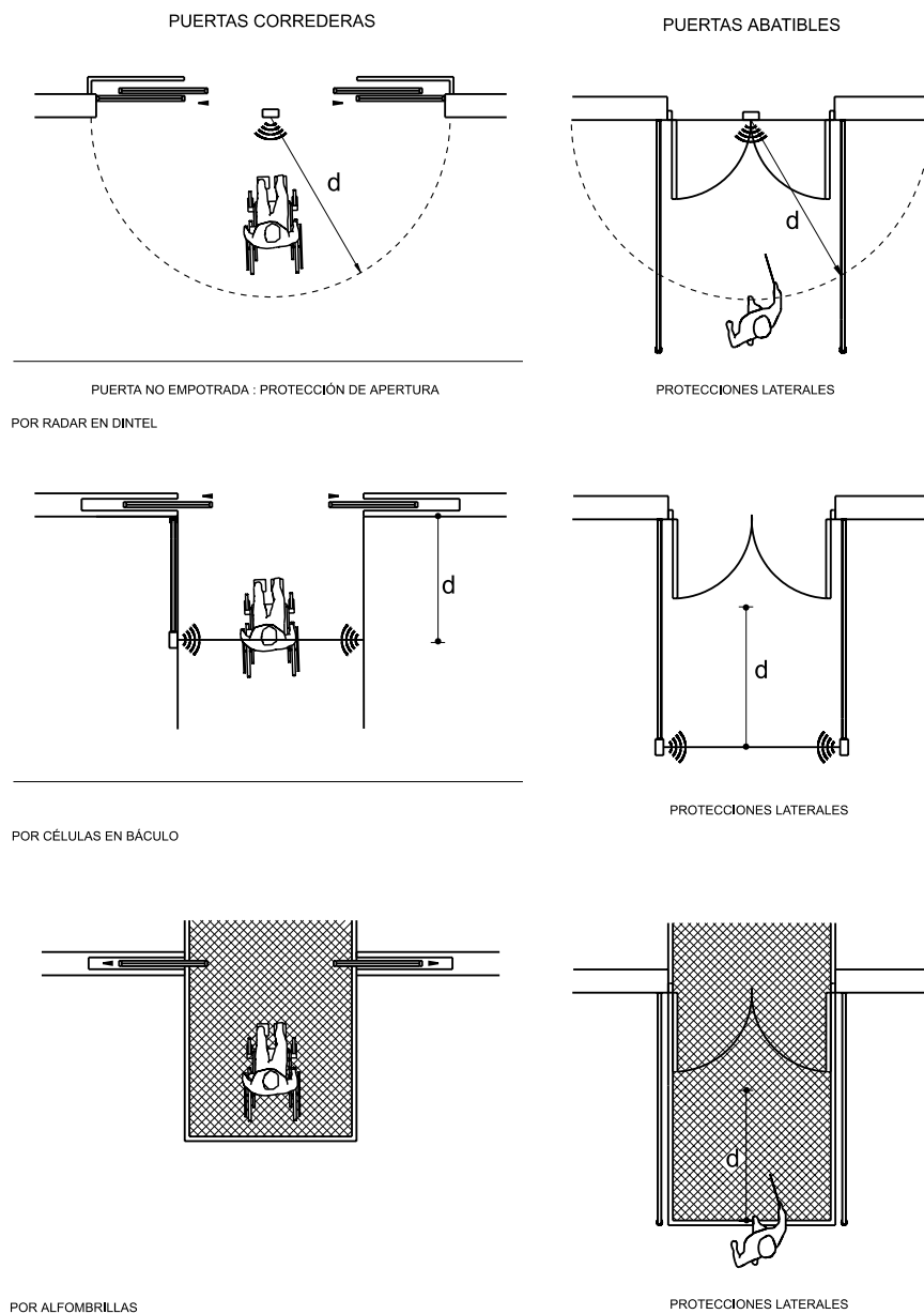
Figura 68.- Puertas automáticas
