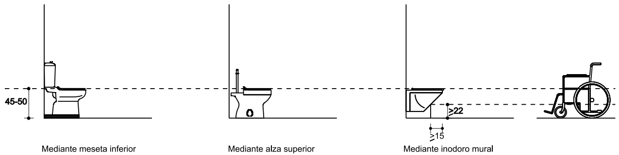
Figura 40.- Altura óptima del asiento del inodoro. Cotas en cm
