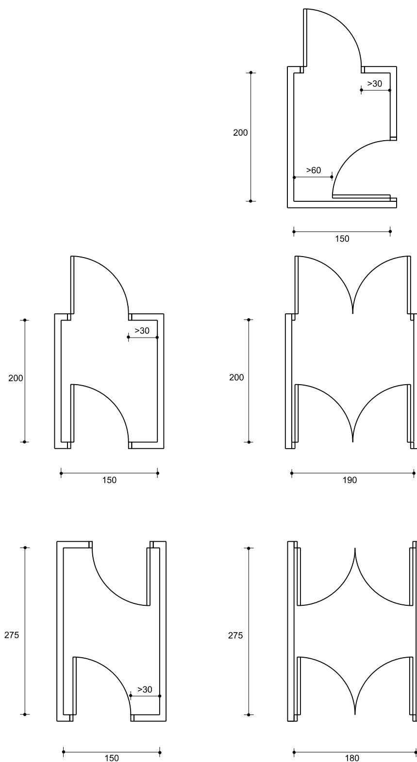
Figura 17.- Vestíbulos. Dimensiones mínimas. Cotas en cm
