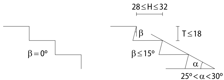
Figura 23.- Trazado de peldaños. Cotas en cm
