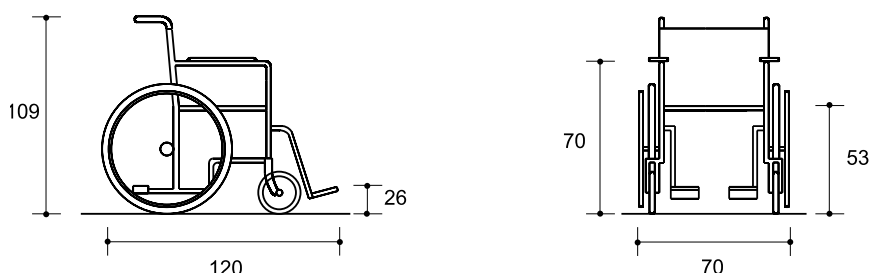
Figura 5.- Dimensiones principales de la silla de ruedas. Cotas en cm
